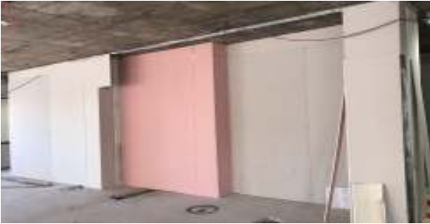
TABIQUE DE ROCA DE YESO - ESTRUCTURA Y 1 PLACA
