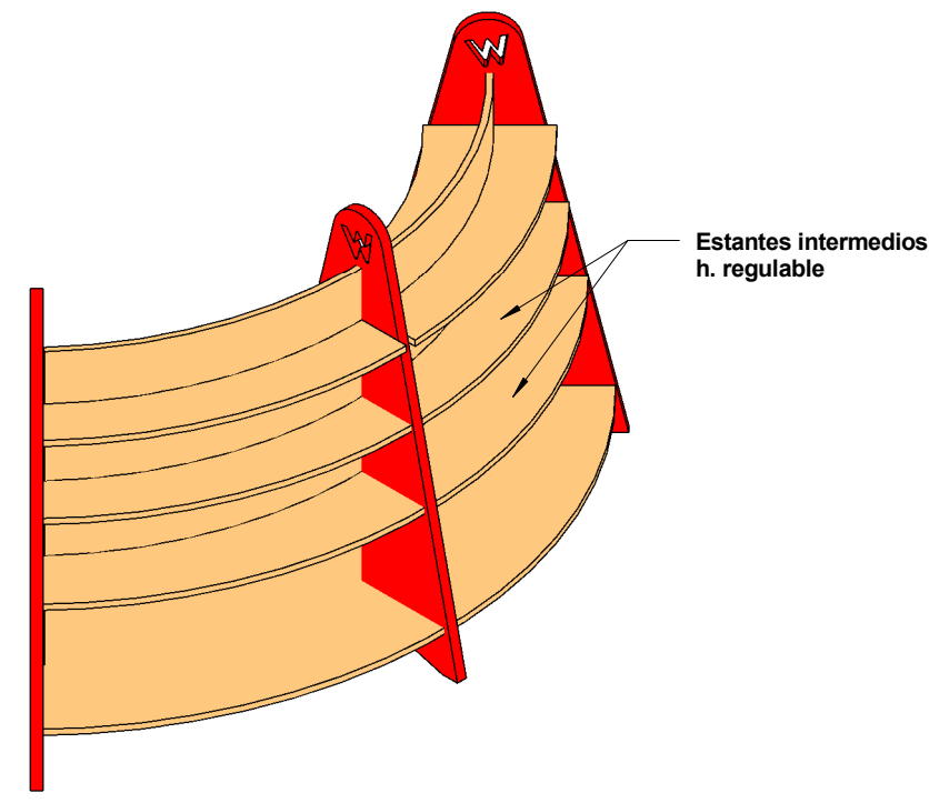
AXONOMETRÍAS
