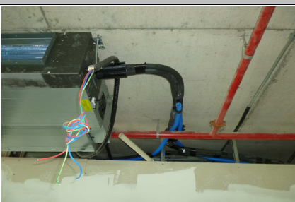
Instalación de aire acondicionado
