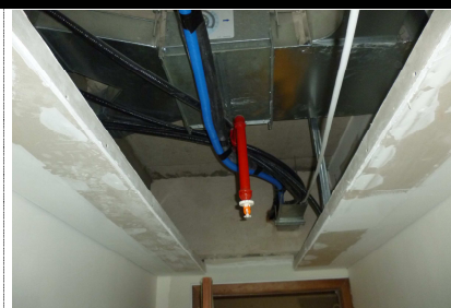
Instalación de extinción de incendio
