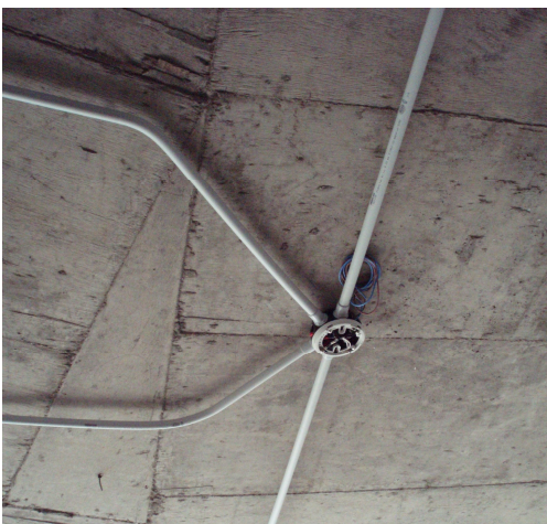
TENDIDO CAÑERIA DETECCION INCENDIO PISOS 5 Y 6
