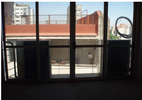
INSTALACION UNIDADES CONDENSADORAS EN BALCONES PISOS 07 -08
