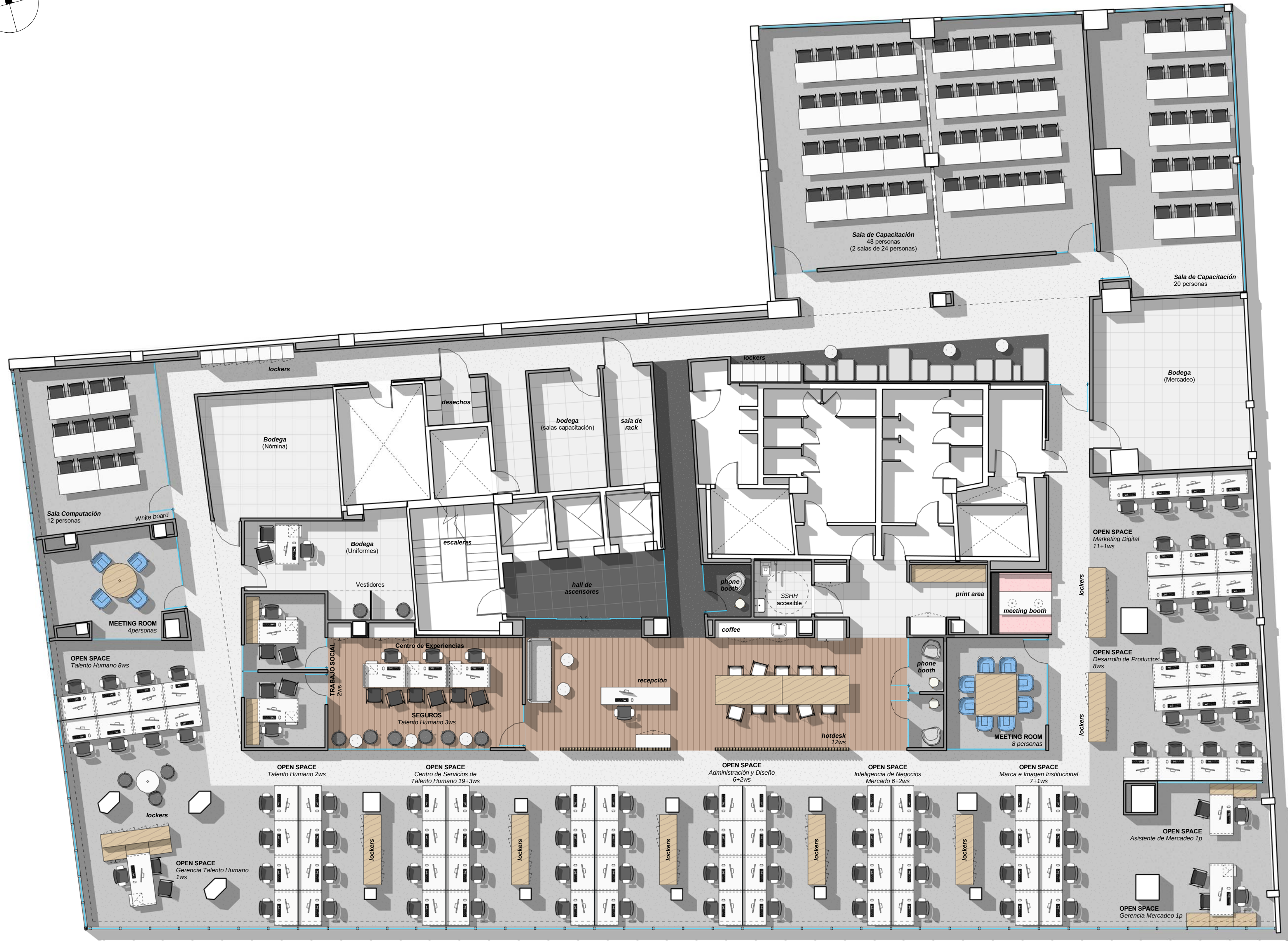
Layout P6 1 : 100
