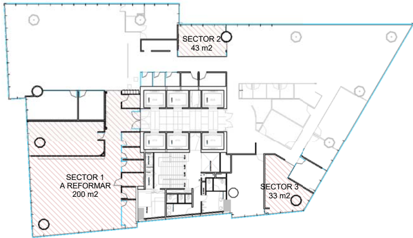
PLANTA UBICACIÓN 1:500 PISO 7
