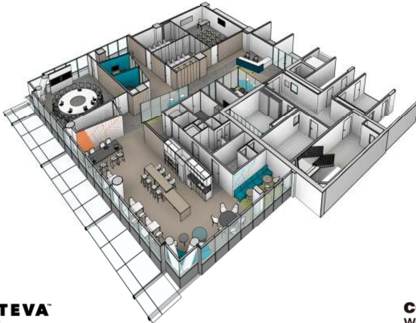
AXONOMETRIA
