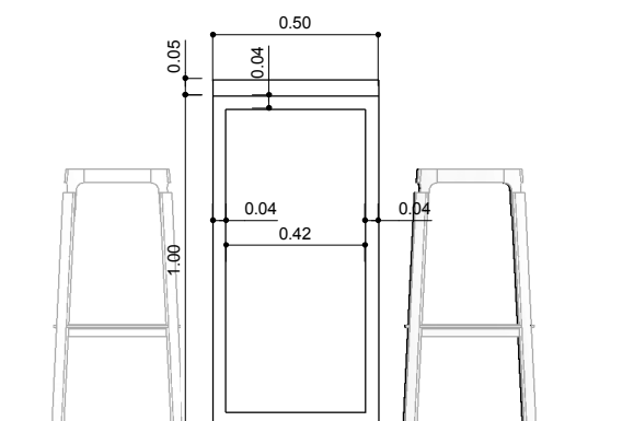
CORTE CB2 BARRA VISTA TRANSVERSAL
