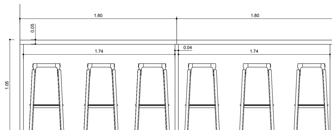
CORTE CB1 BARRA VISTA LONGIUDINAL
