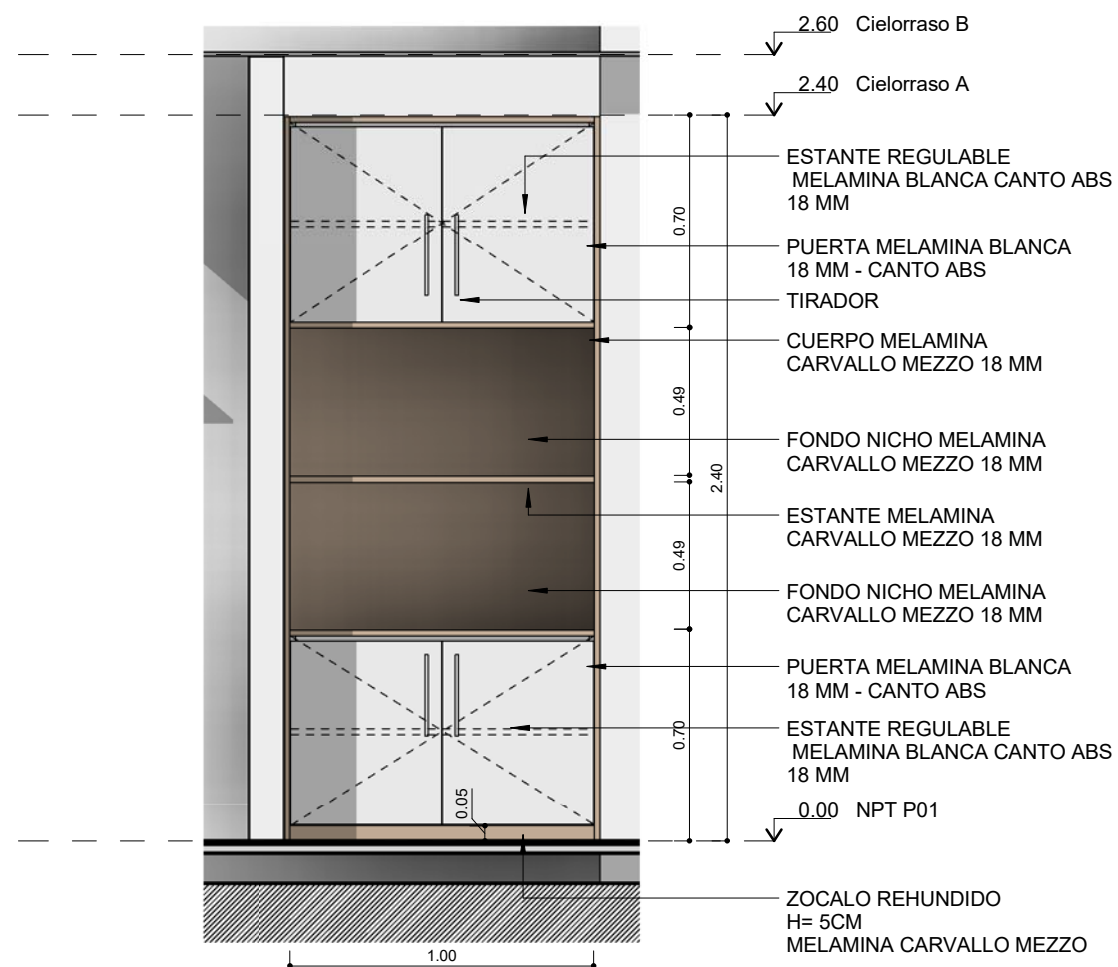
VISTA FRENTE 1 : 25
