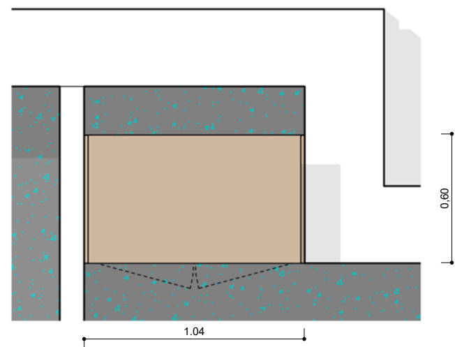
PLANTA 1 : 25
