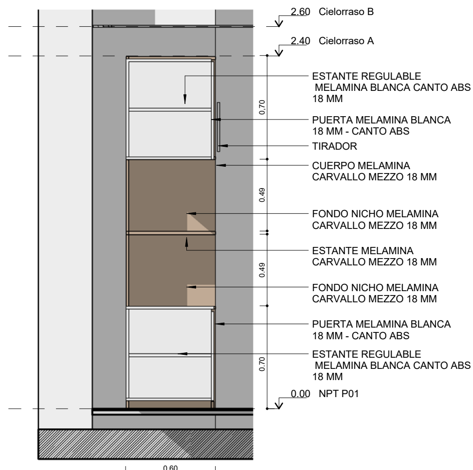
CORTE 1 : 25
