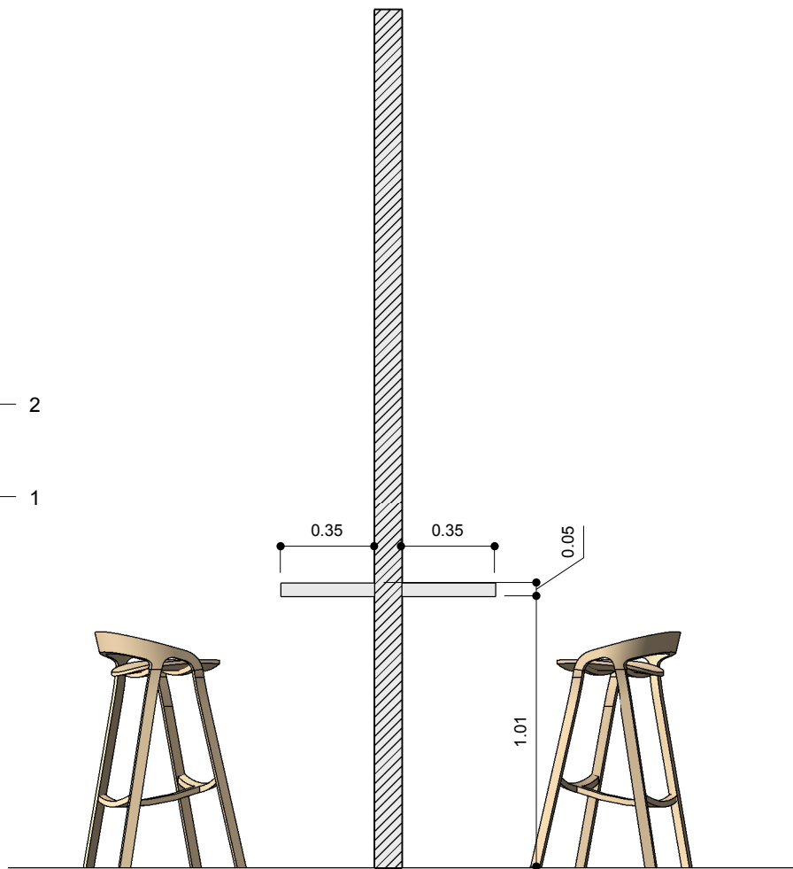
Corte
