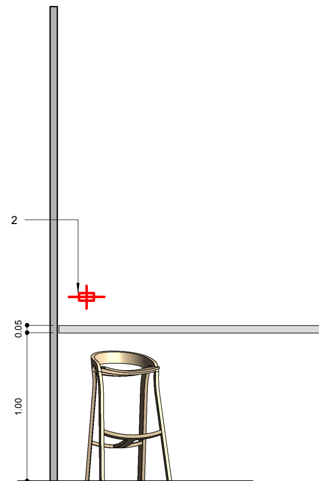
Corte
