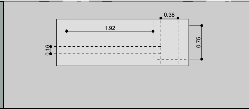
LOGO CORPÓREO 2 Acero Inoxidable esmerilado - Calidad 304 - 1mm espesor Fijación con pernos Cant.: 1
