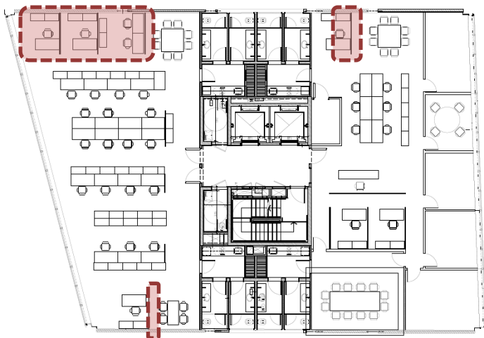
SEGUNDO PISO
