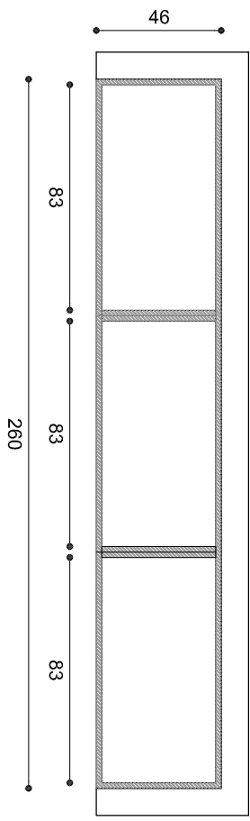
PLANTA MUEBLE ARCHIVO / Me01 CANT: 2
