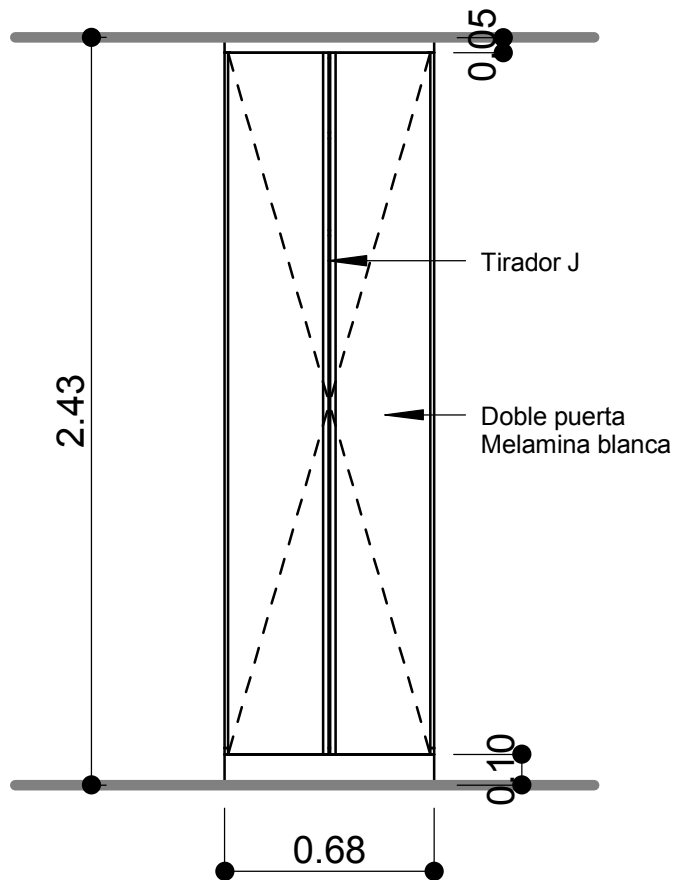
VISTA EXTERIOR
