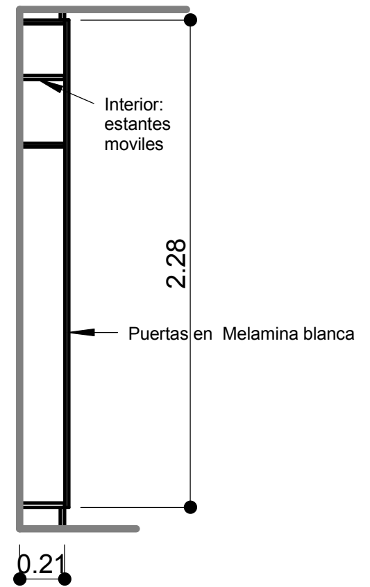
CORTE
