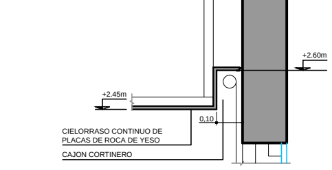
DETALLE 3
