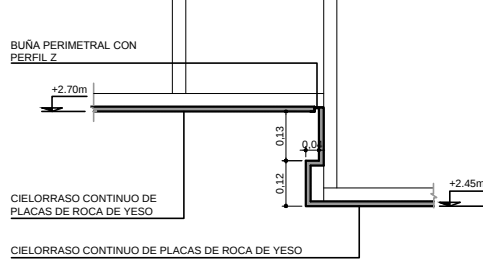
DETALLE 2
