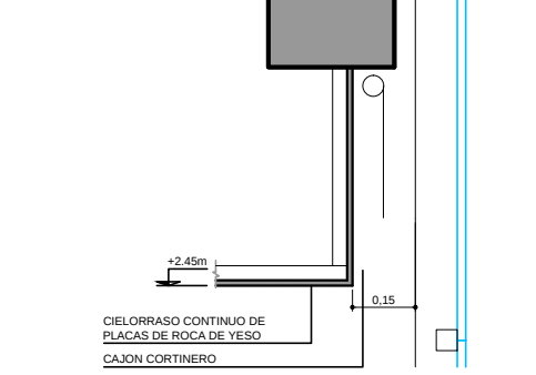
DETALLE 4
