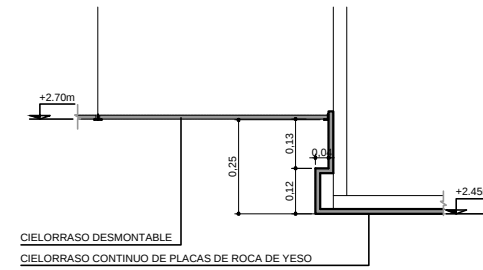
DETALLE 1
