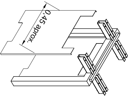
Axonometrica
