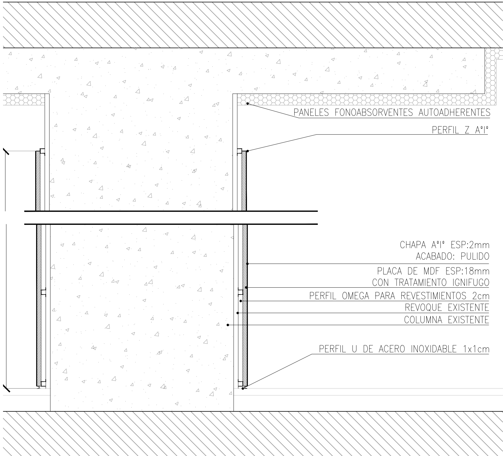
C5-CORTE ESC. 1:10
