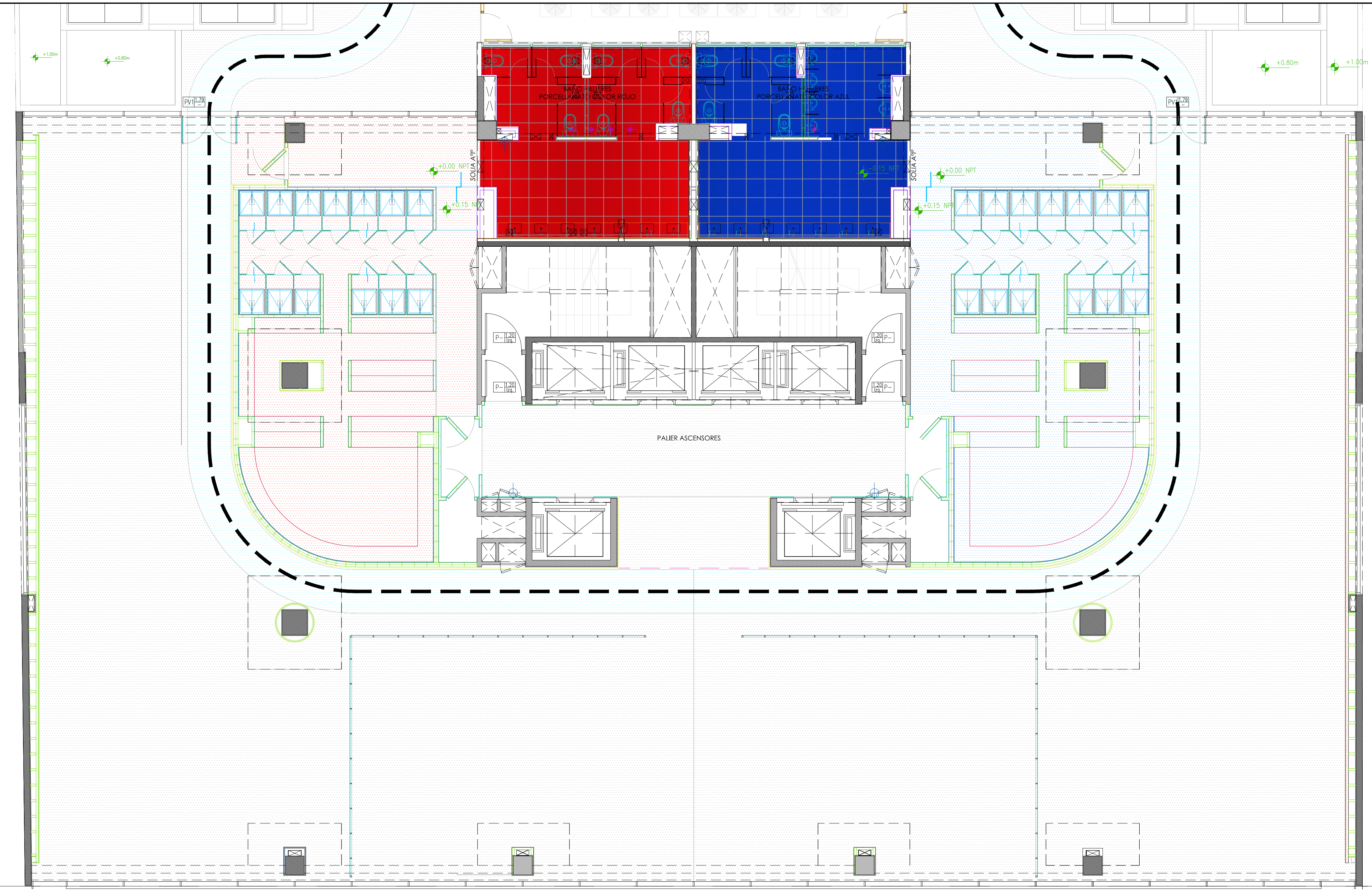
3° PISO PLANTA DE SOLADOS INTERIORES
