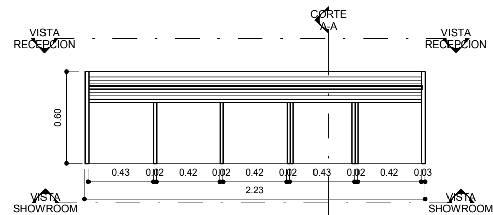
PLANTA 1 : 25
