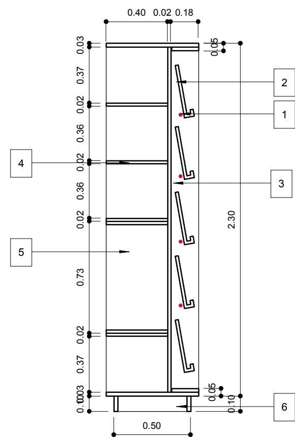
CORTE A-A 1 : 25
