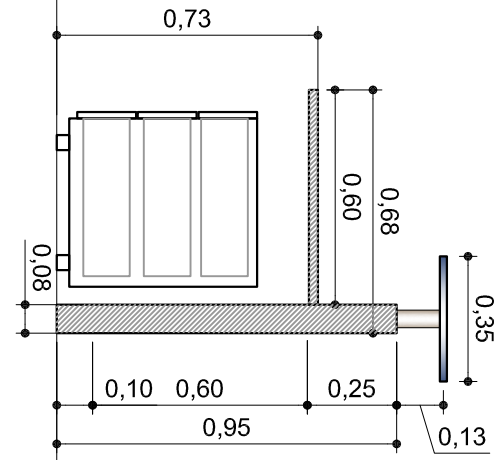
CORTE A-A
