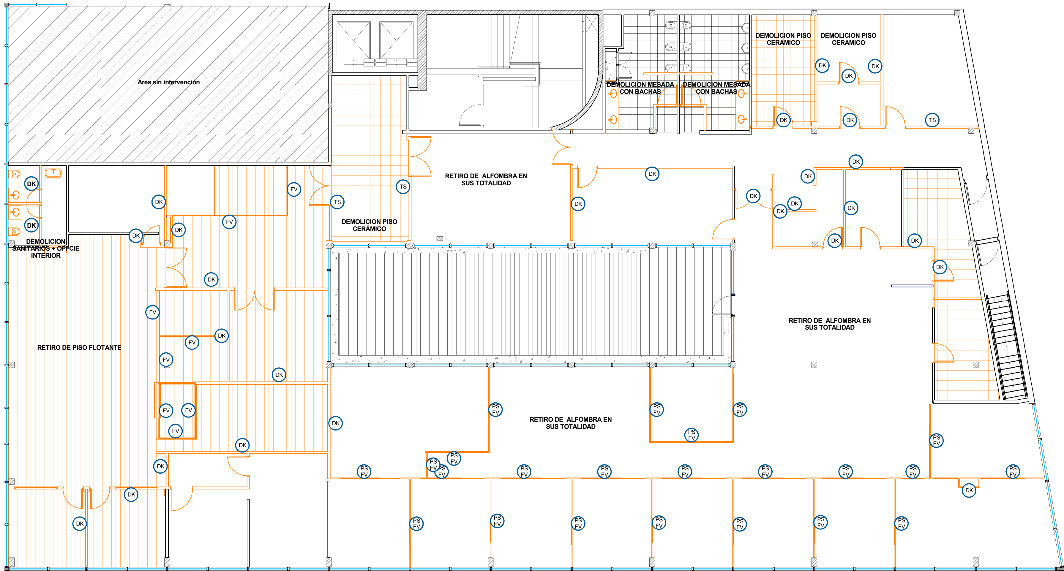
Tabiquería Demolición 1 : 100
