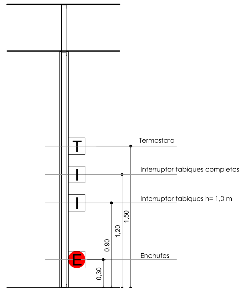
Corte basico
