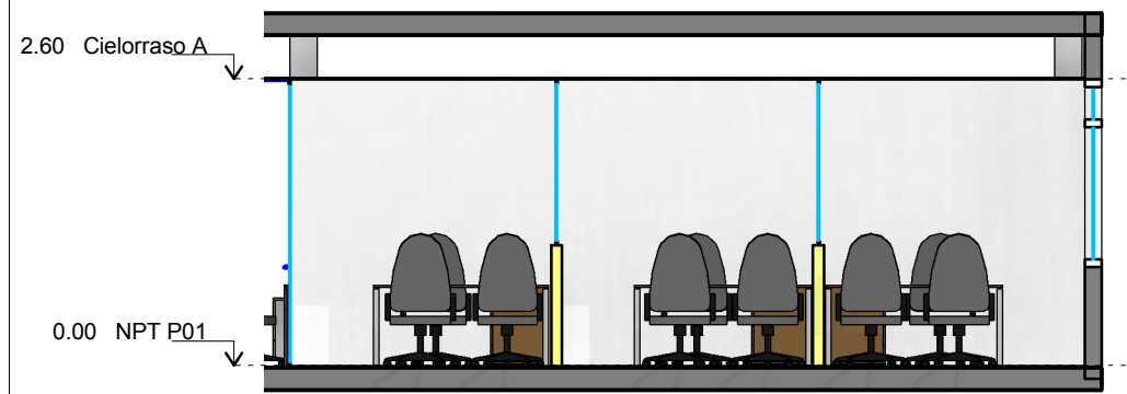
Area Finanzas 1 : 75
