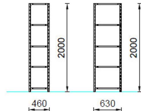
ELEVACION LATERAL
