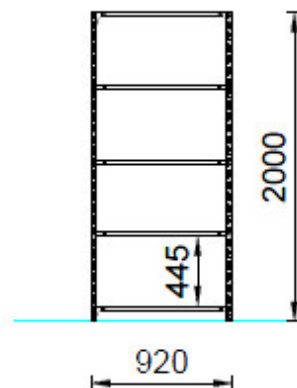
ELEVACION FRONTAL
