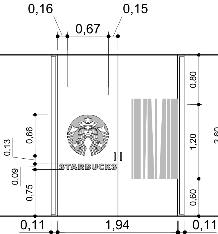
Elevacion 10, Puerta Acceso Esc 1:25
