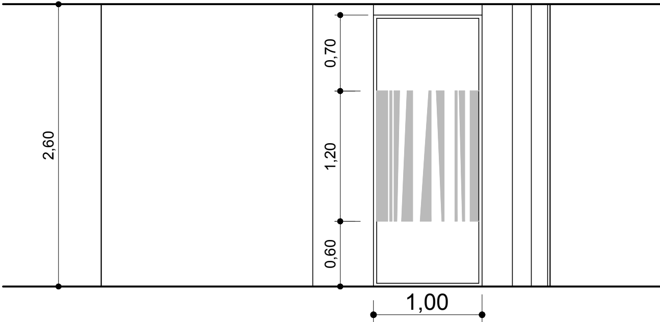
Elevacion 7 Break Coffee Esc 1:25
