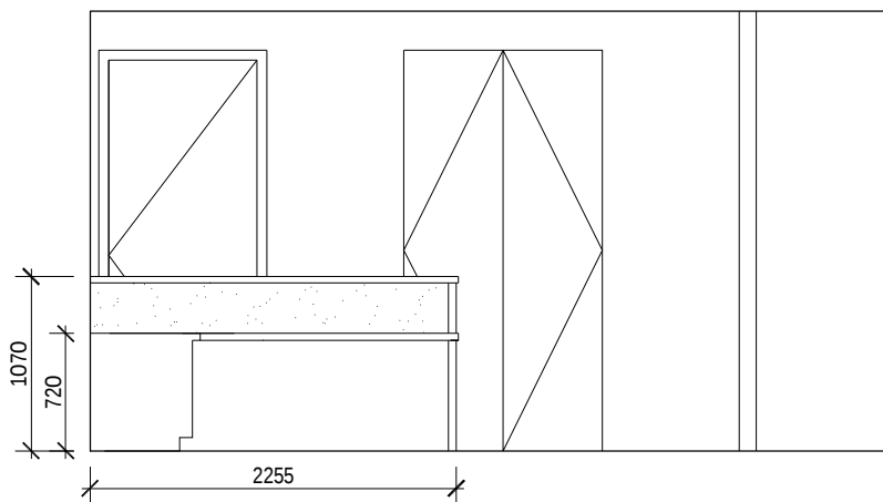
3 ELEVATION SCALE: 1:50
