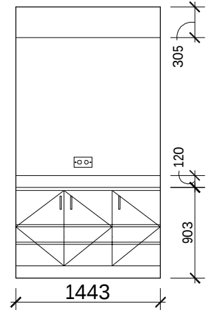
5 ELEVATION SCALE: 1:50
