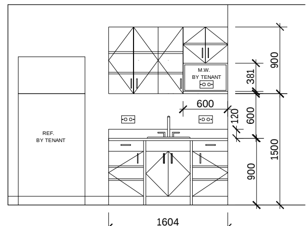
ELEVATION SCALE: 1:50
