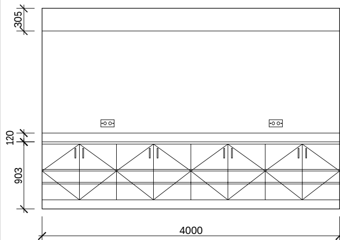
6 ELEVATION SCALE: 1:50
