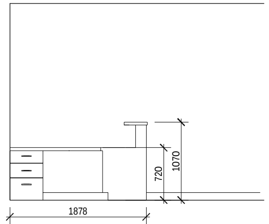
2 ELEVATION SCALE: 1:50
