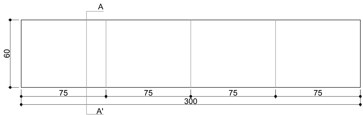
Planta mueble sala de reuniones
