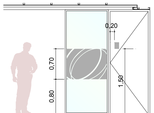
Elevacion Oficinas Oriente
