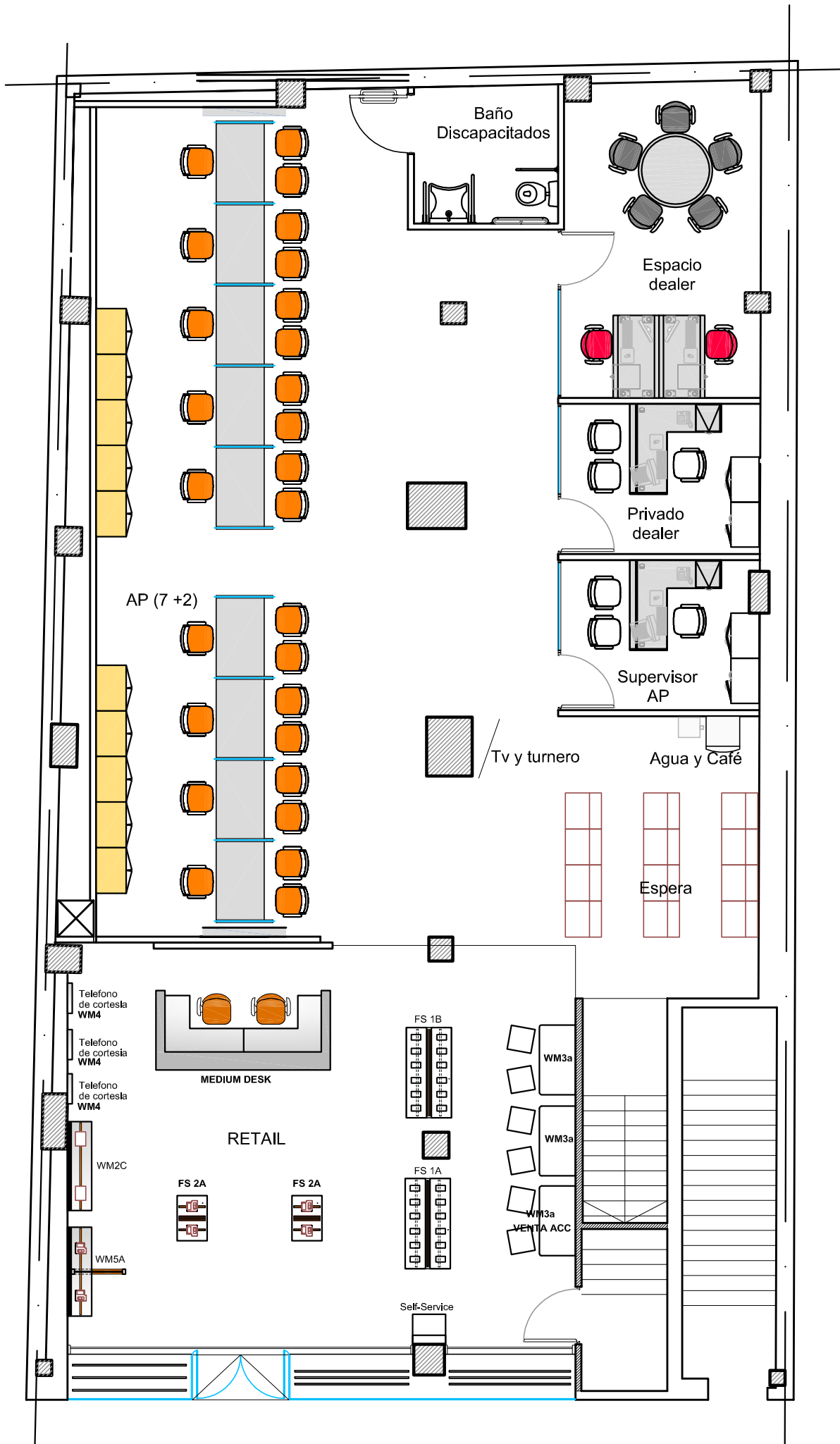
PLANTA BAJA
