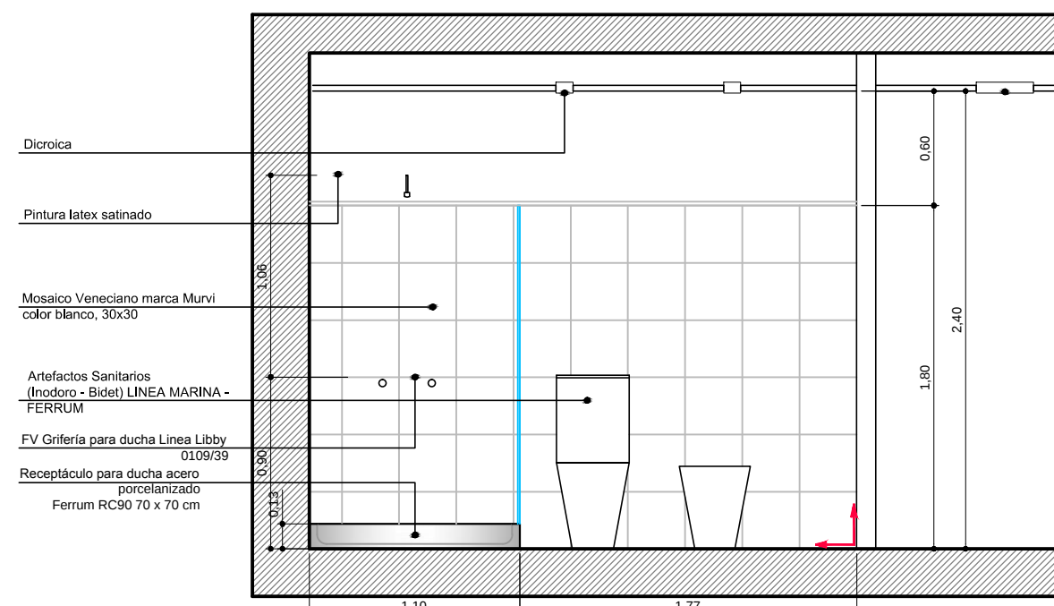
CORTE TRANSVERSAL A-A
