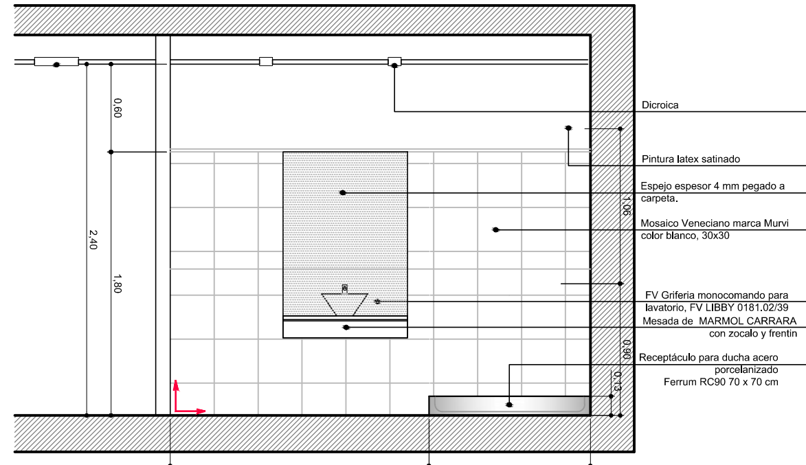
CORTE TRANSVERSAL B-B
