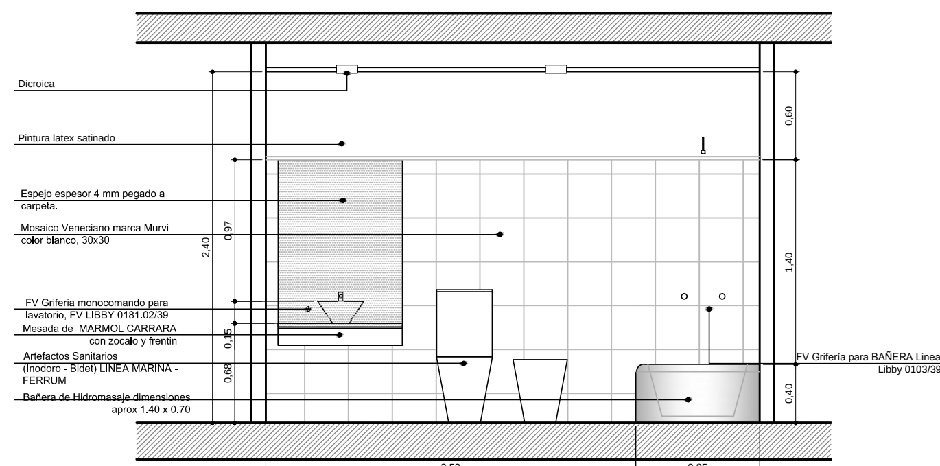
CORTE TRANSVERSAL A-A
