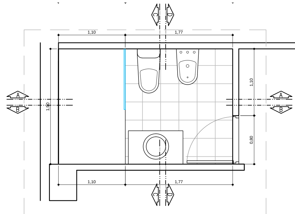
PLANTA ARQUITECTURA
