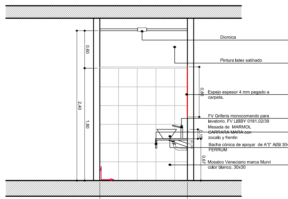
CORTE TRANSVERSAL C-C
