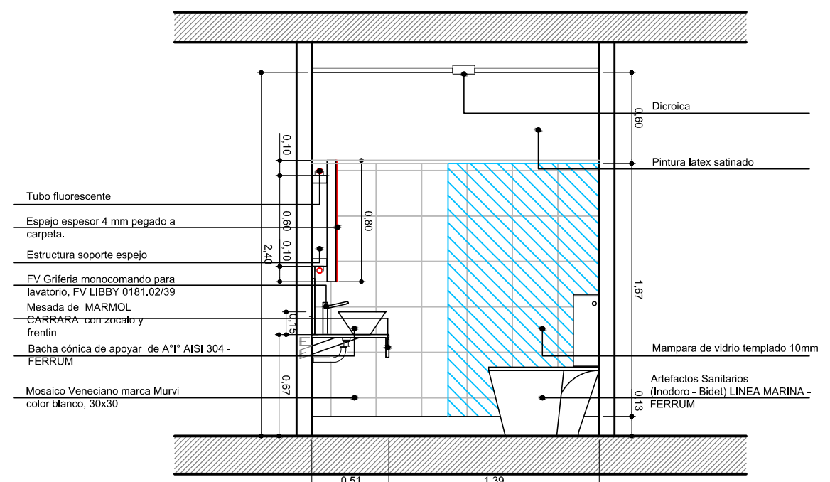
CORTE TRANSVERSAL C-C
