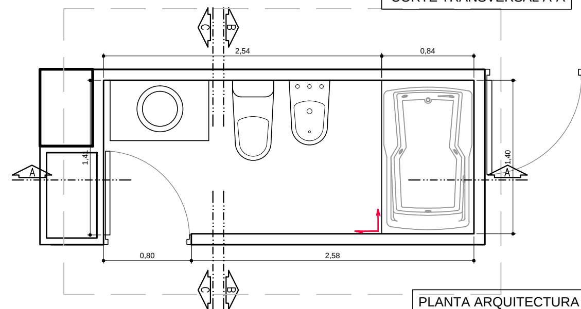
PLANTA ARQUITECTURA
