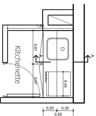
PLANTA MUEBLE KICHENETTE
