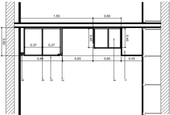
CORTE A-A
