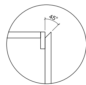
DETALLES TIRADOR TIPO CAVA ESC 1/5
