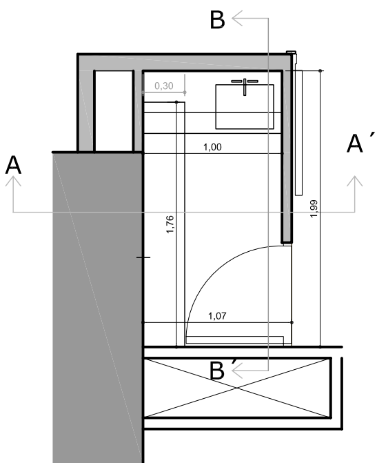
PLANTA MUEBLE. esc 1:20
