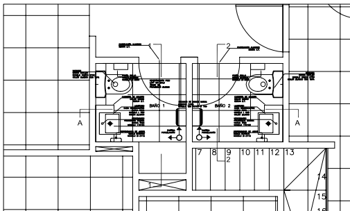
PLANTA BAÑO 1 Y 2 ESCALA 1:50
