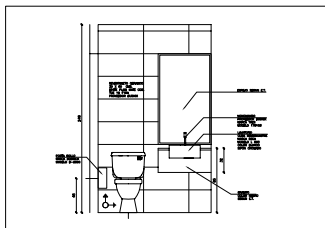
CORTE 2-2 BAÑO 2 ESCALA 1:20
