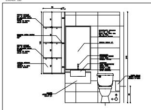
CORTE 1-1 BAÑO 1 ESCALA 1:20
