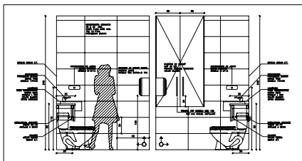
CORTE A-A BAÑO 1 Y 2 ESCALA 1:20
