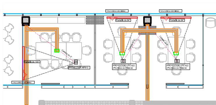
PD-2 SALA DE REUNIONES SECTOR ARGENTINA ESC. 150
