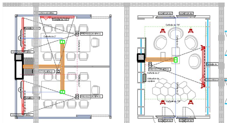
PD-1 SALA DE REUNIONES SECTOR LATAM ESC. 150
