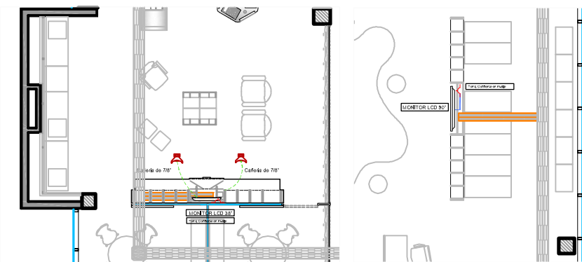
PD-3 SALA DE EXPERIMENTACION SECTOR ARGENTINA ESC. 150
