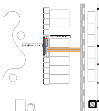
PD-4 MUEBLE EXPOSICION PRODUCTOS ARGENTINA ESC. 150
