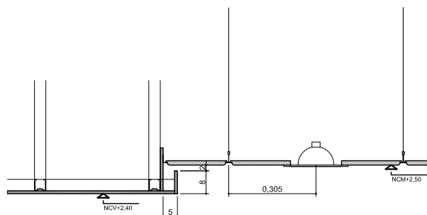
CORTE 1 ESC: 1/10
