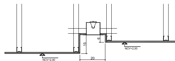
CORTE 2 ESC: 1/10
