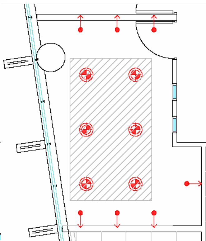
CIELO / ILUMINACIÓN
