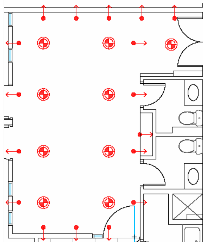
CIELO / ILUMINACIÓN
